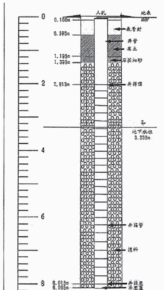
監測井結構圖
