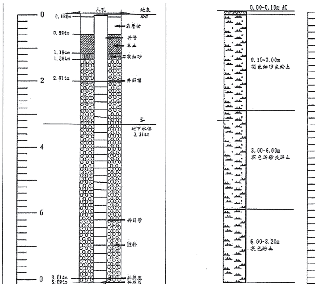
監測井結構圖
