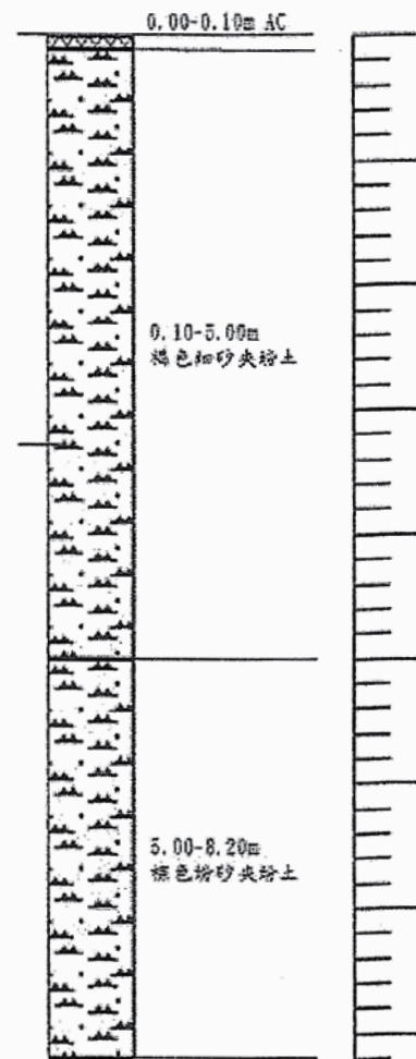
地質剖面圖
