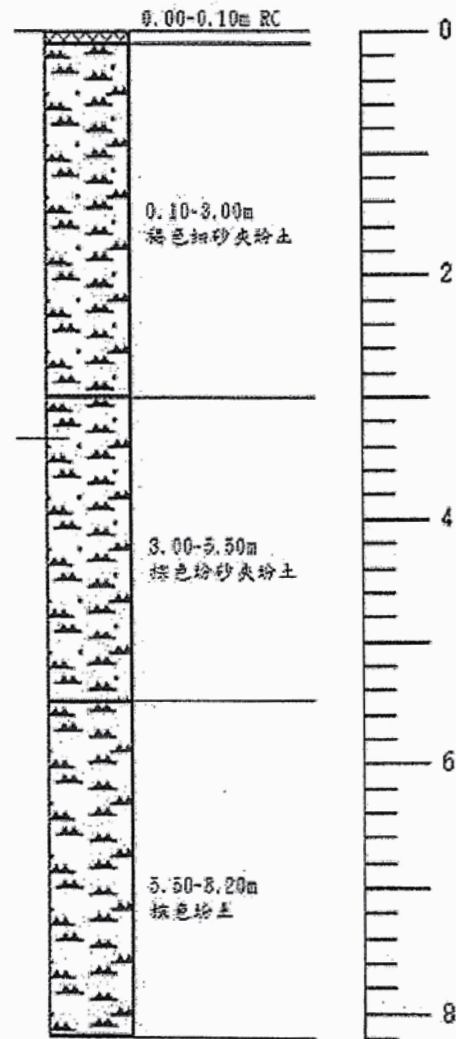
地質剖面圖
