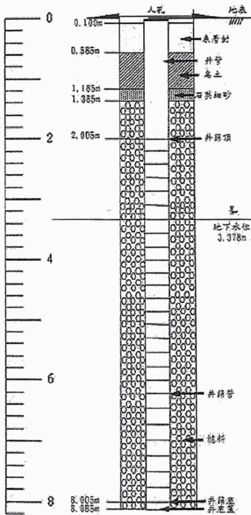
監測井結構圖
