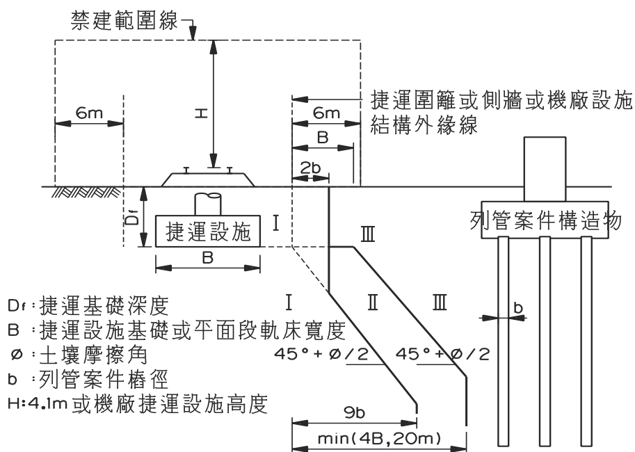
圖二十九 列管案件為基樁之分級規範界線圖 【地面段、出土段、機廠直接基礎及筏式基礎適用】
