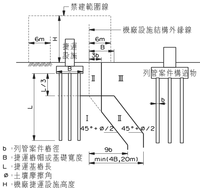
圖三十一 列管案件為基樁之分級規範規範圖【機廠樁基結構適用】
