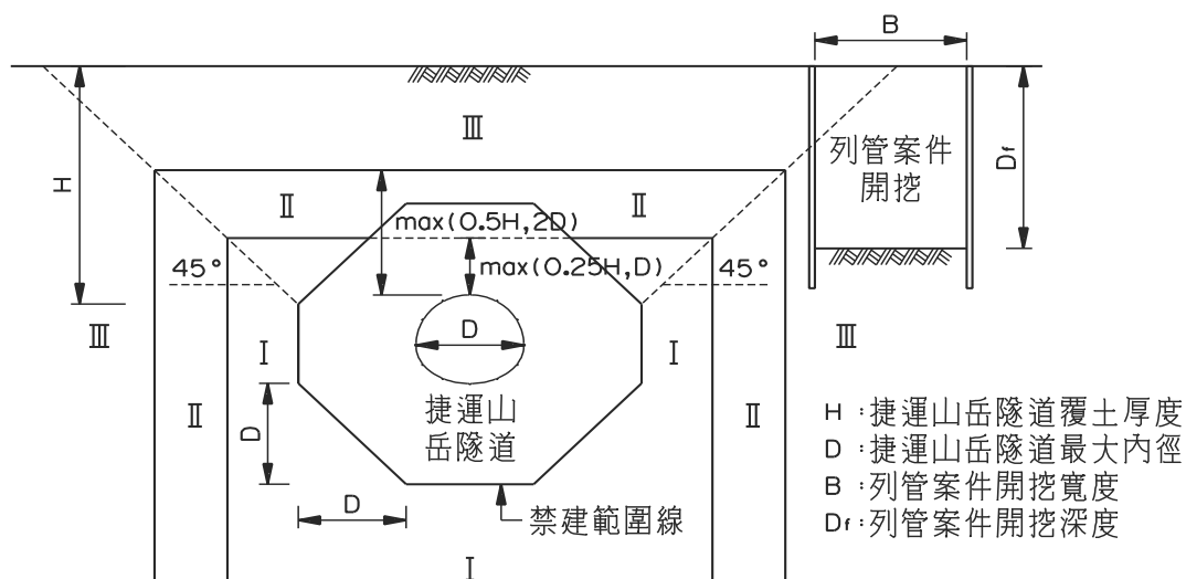
圖六 列管案件為明挖工程之分級規範界線圖【山岳隧道段適用】
