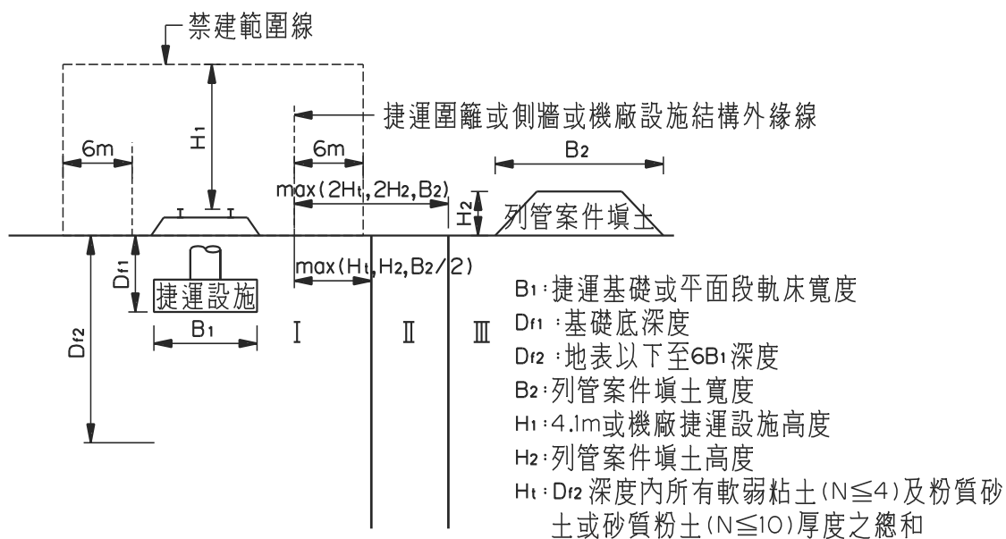
圖十七 列管案件為填土工程之分級規範界線圖
