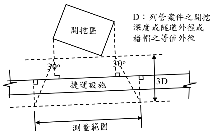
圖一 捷運設施在開挖區側邊之現況測量範圍(平面圖)
