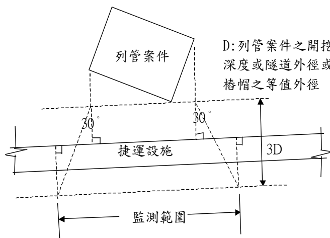
圖一 捷運設施上之監測儀器佈設範圍平面圖 (超出 3D 範圍之捷運設施可不必裝設)
