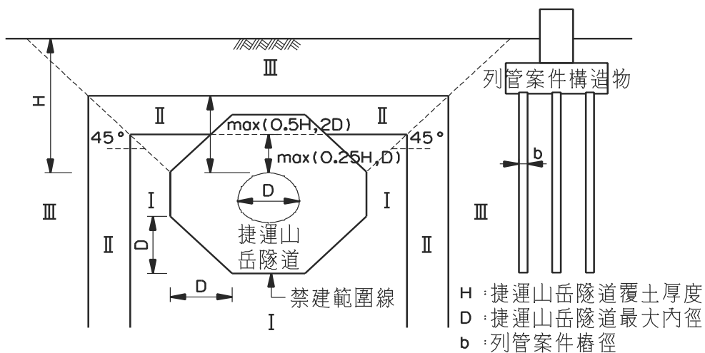
圖三十二 列管案件為基樁之分級規範界線圖【山岳隧道段適用】
