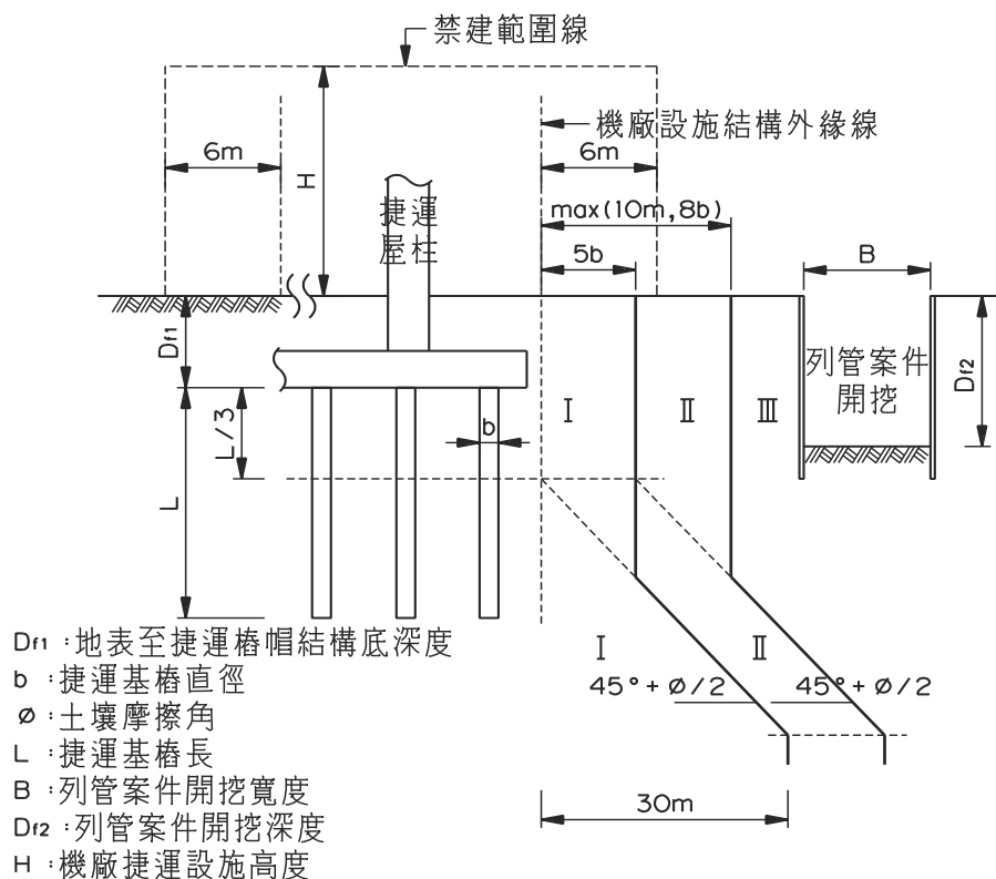
圖五 列管案件為明挖工程之分級規範界線圖【機廠樁基結構適用】
