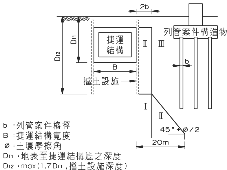
圖二十八 列管案件為基樁之分級規範界線圖【明挖隧道、車站及管幕隧道段適用】
