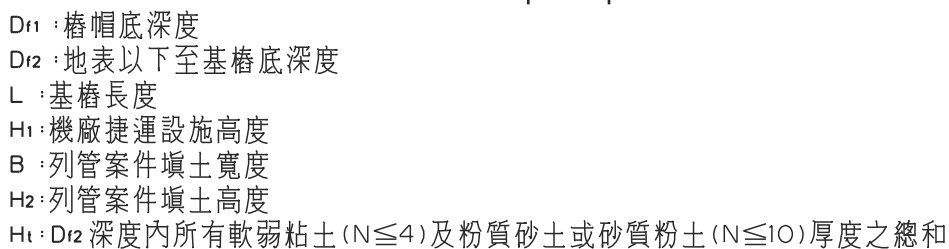
圖十九 列管案件為填土工程之分級管制界線圖【機廠樁基結構適用】
