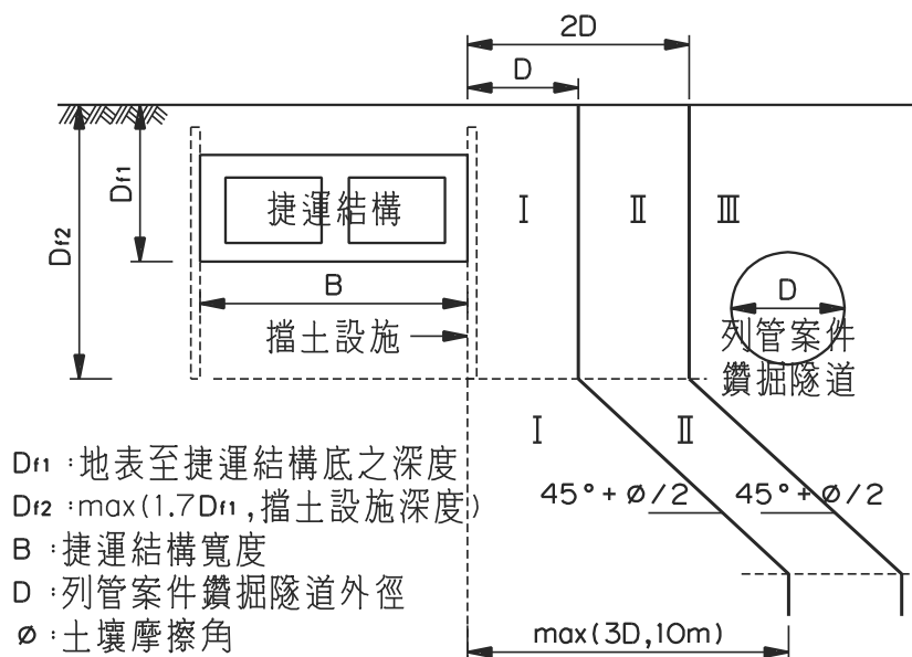
圖十 列管案件為鑽掘隧道之分級規範界線圖【明挖隧道、車站及管幕隧道段適用】
