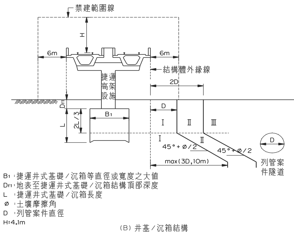
圖二十三 列管案件為山岳隧道之分級規範界線圖【高架段(樁基結構、井基/沉箱結構)適用】
