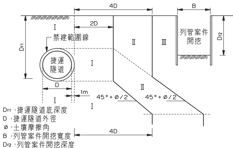
圖一 列管案件為明挖工程之分級規範界線圖【潛盾隧道段(含隧挖段)適用】
