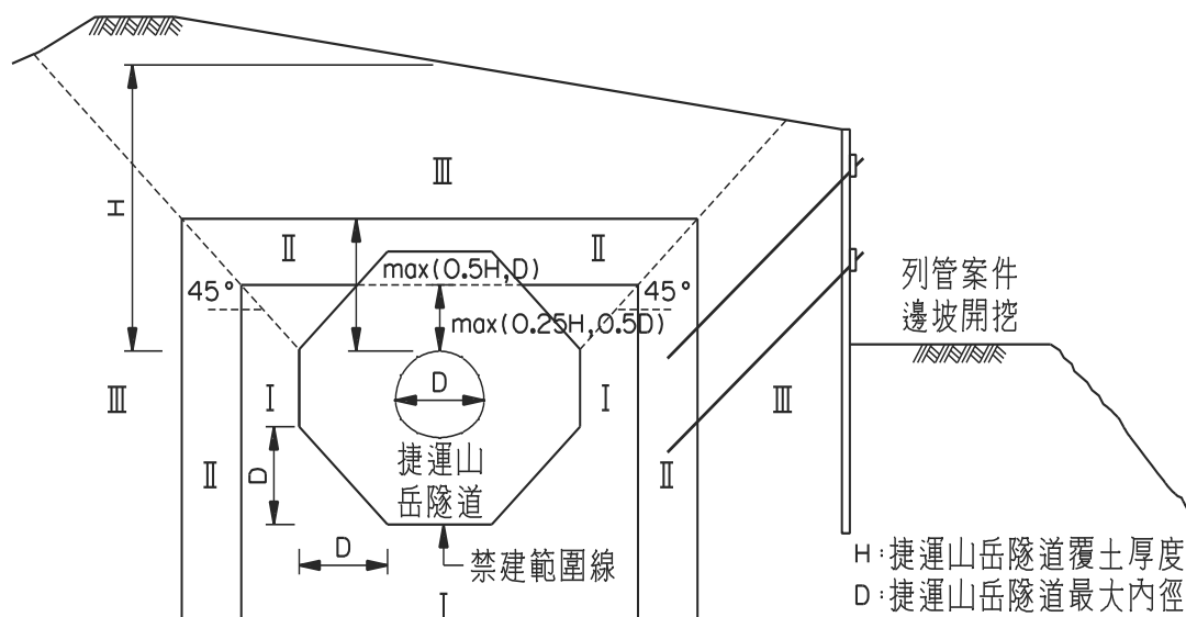
圖七 列管案件為錨固邊坡開挖工程之分級規範界線圖【山岳隧道段適用】
