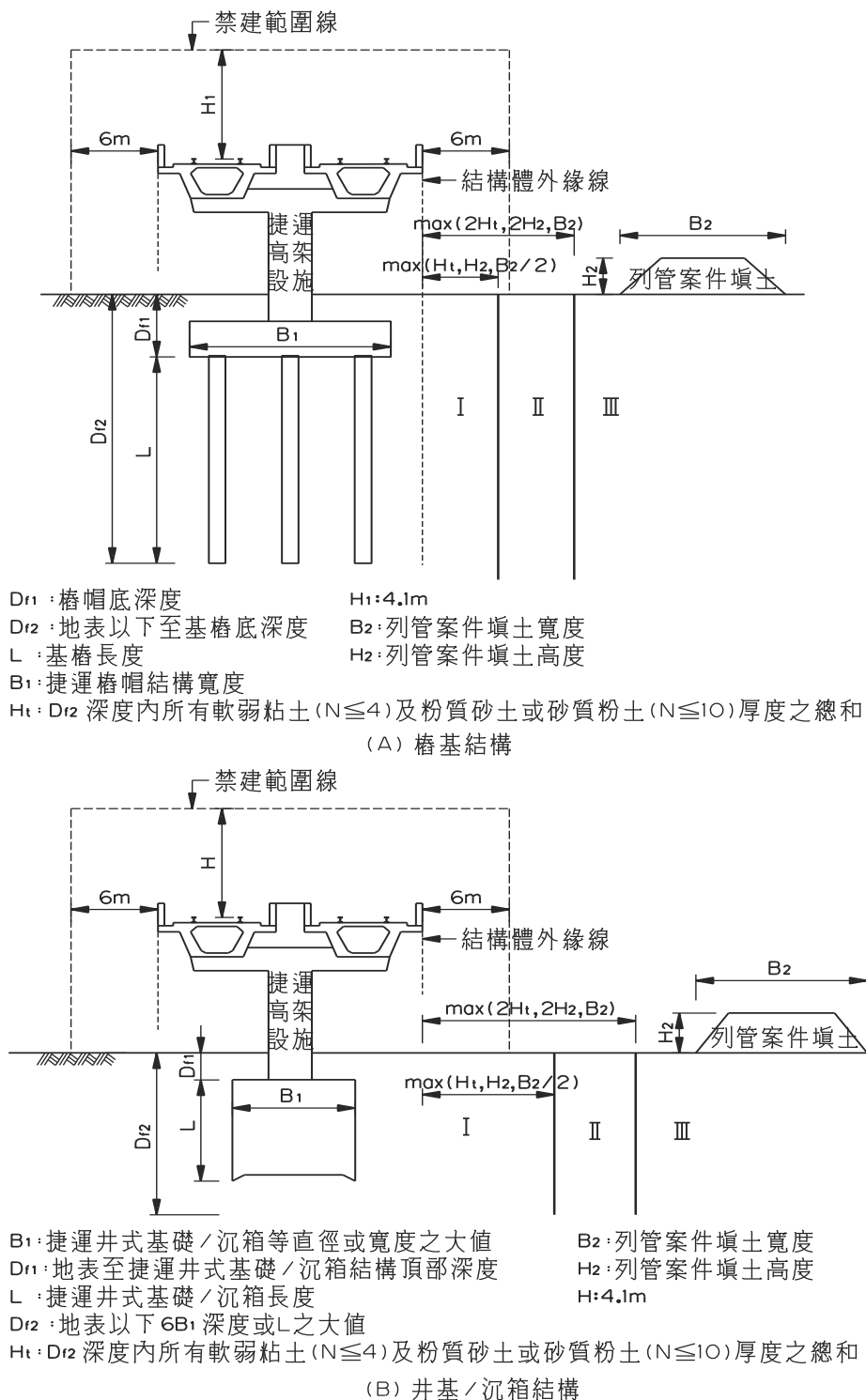
圖十八 列管案件為填土工程之分級管制界線圖【高架段(樁基結構、井基/沉箱結構)適用】
