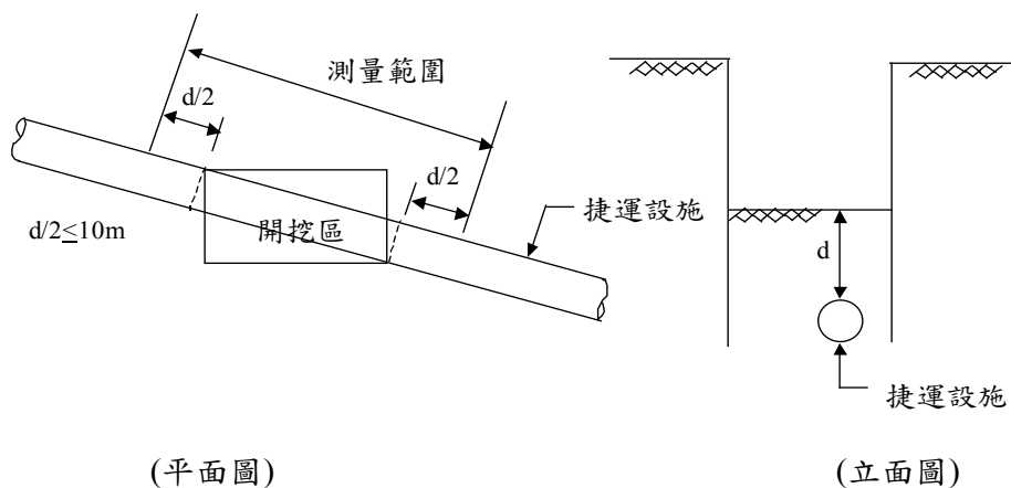
圖二 捷運設施在開挖區下方之現況測量範圍
