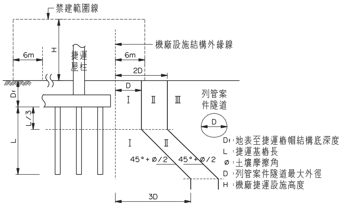
圖二十四 列管案件為山岳隧道之分級規範界線圖【機廠樁基結構適用】
