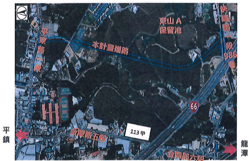
圖 1 工程範圍圖
