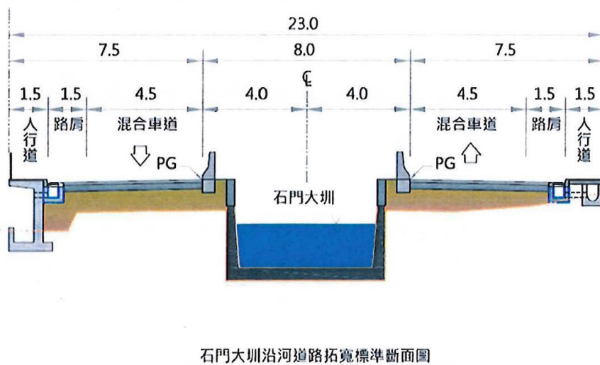
圖 5 標準断面配置圖
