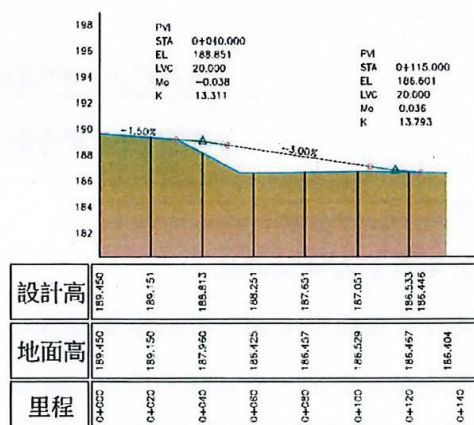
圖 4 石門大圳道路坡度順修示意圖
