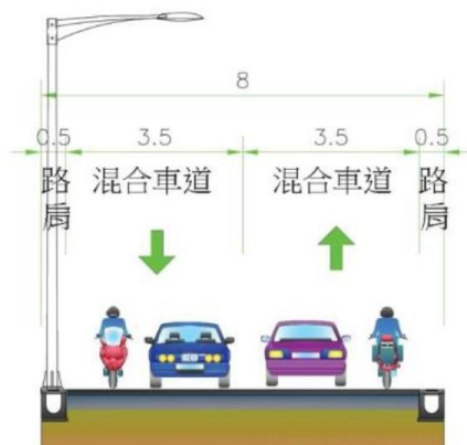
圖 2-桃園市「平鎮區新興路 179 巷 9 弄（新興路 177 巷 24 弄至義興街）道路新闢工程」道路配置
