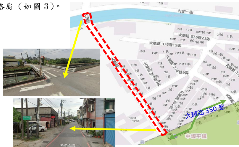
圖 2-桃園市「中壢區大華路（內定一街至大華路 350 巷）道路拓寬工程」計畫內容
