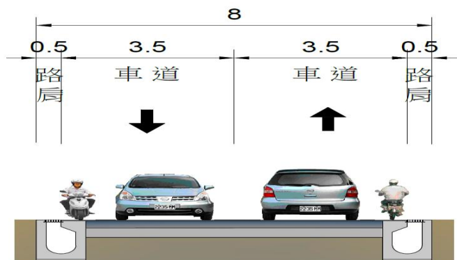
圖 3-桃園市「中壢區大華路（內定一街至大華路 350 巷）道路拓寬工程」道路配置圖
