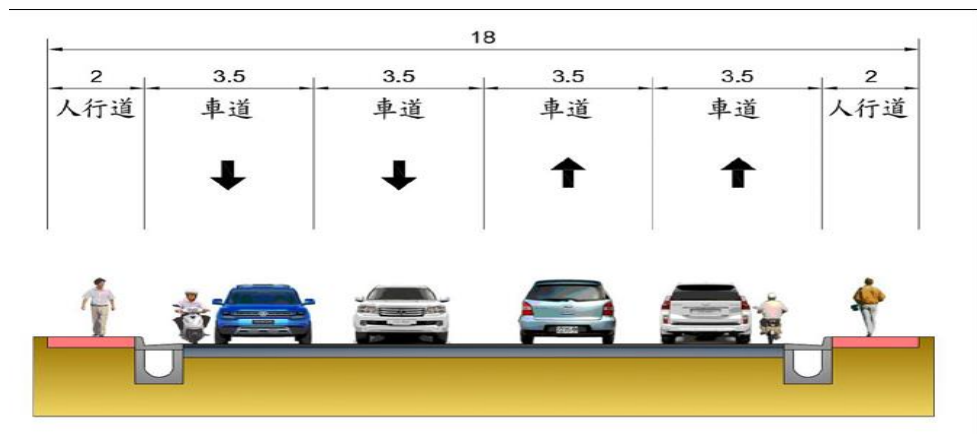
圖 2 道路配置圖
